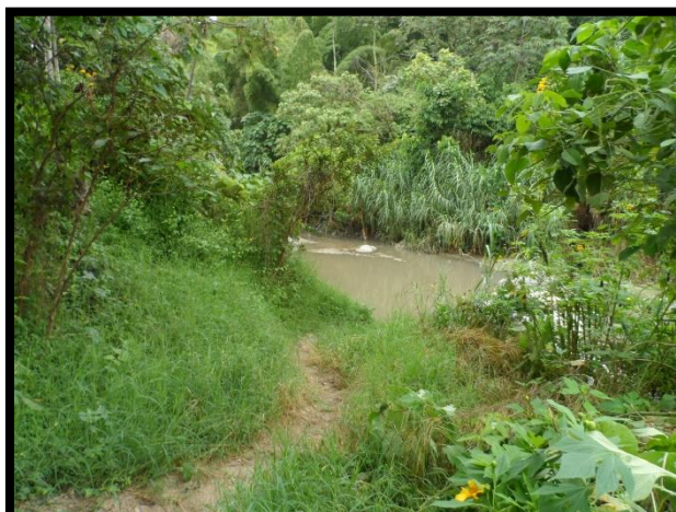
Imagen 28. Aluviones y terrazas de la quebrada Aguas Frías. Fuente: Grupo Formalización Minera 2017.
