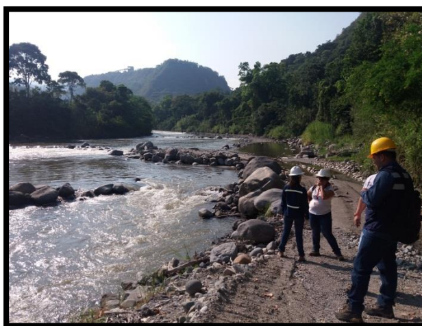
Imagen 47. Frente de explotación Depósitos del río Coello. Fuente: Grupo Formalización Minera 2017.
