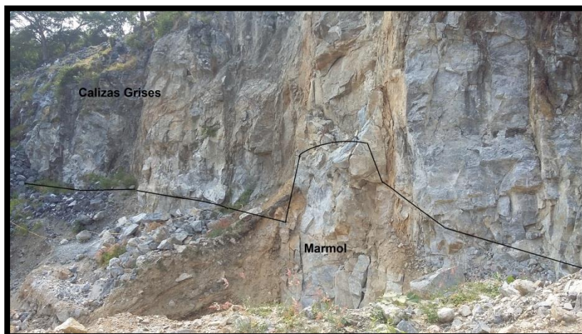
Imagen 86. Unidades geológicas correspondientes a la Formación Payandé (Rpc – Rpm). Fuente: Grupo Formalización Minera 2017.
